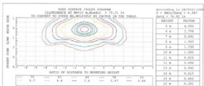
แผนภาพแสดงแสงสว่างเท่าบนผิวถนน
