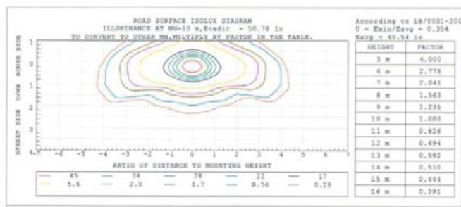
แผนภาพแสดงเส้นความส่องสว่างเพาบนถนน
