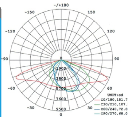
แผนภาพแสดงเส้นความส่องสว่างเพาบนถนน
